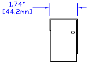
L. END VIEW
